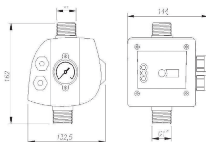
Dimensiones - esquema técnico
